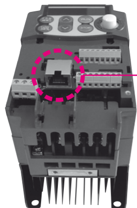
Porta di comunicazione RS-485
